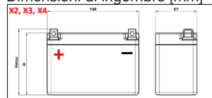
Dimensioni di ingombro [mm]
